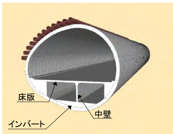
STEP10: 内部構築
