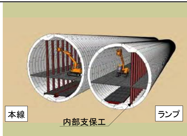
STEP2:内部支保工組立・坑内仮設備工
