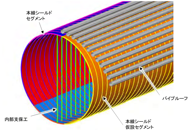
解析モデル(南行)概要
