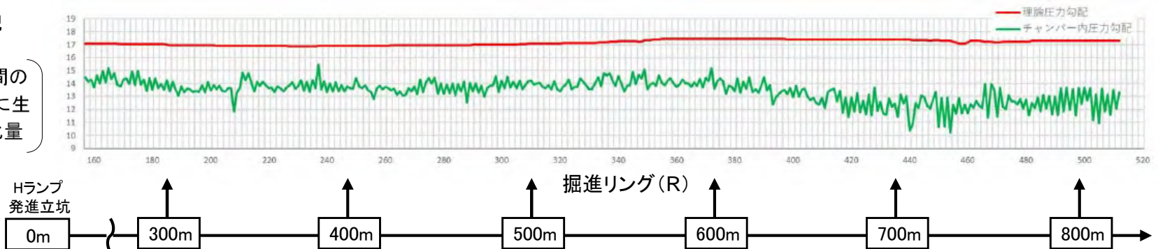
チャンバー内圧力勾配 (kPa/m)
