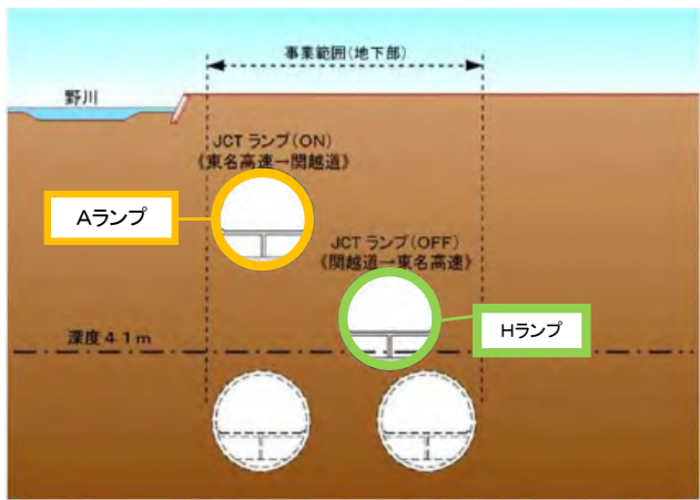
A-A断面
