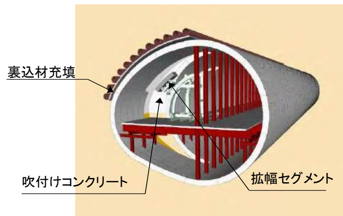
STEP7: 拡幅セグメント設置
