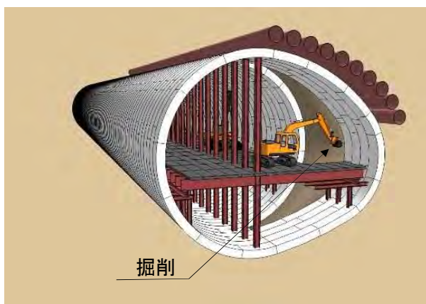
STEP6: 拡幅掘削
