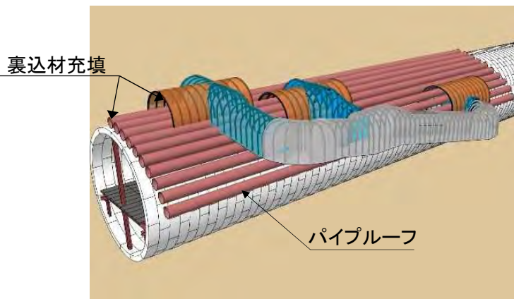
STEP4: パイプルーフ施工
