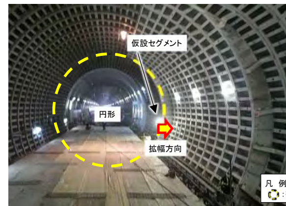
部分拡幅工法 (中央環状品川線大橋連絡路工事の事例)
