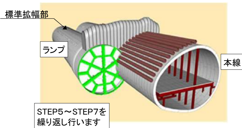
STEP8: 東名側(標準拡幅部)到達
