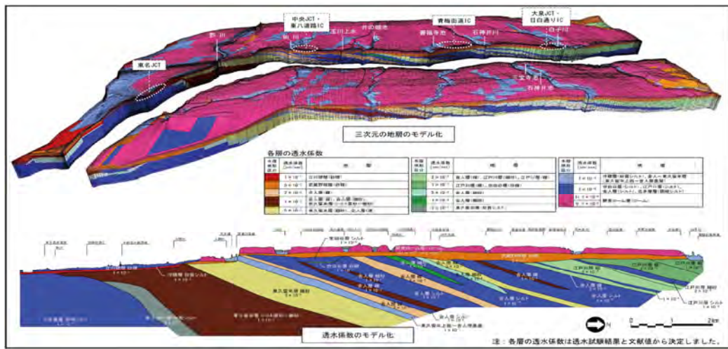
三次元浸透流解析における計算格子モデル 出典：環境影響評価書 資料編（平成19年3月）
