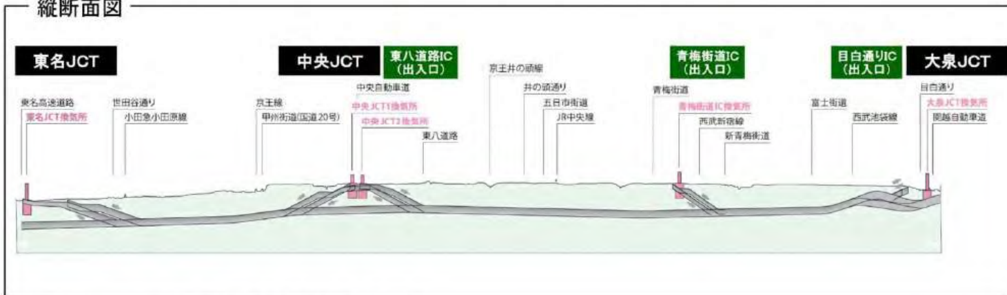
縦断面図
