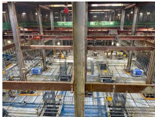
換気所地下工事の坑内 野川上流側を望む (令和6年11月27日)
