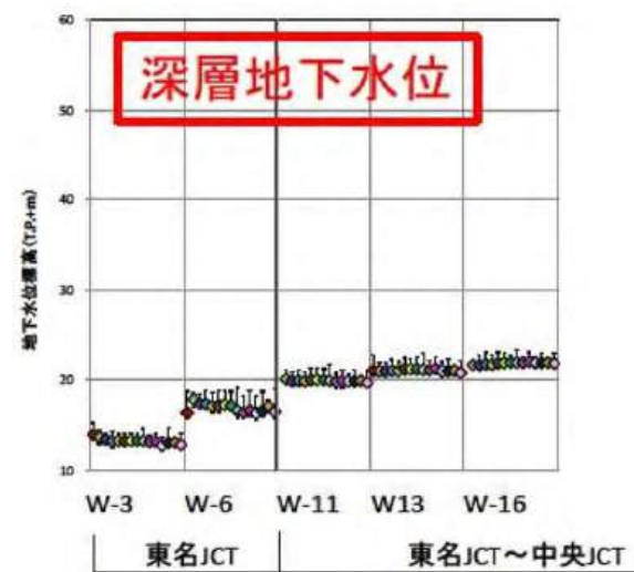
深層地下水位 年間平均値
