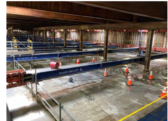
Hランプ函体構築の状況 (令和6年8月28日)
